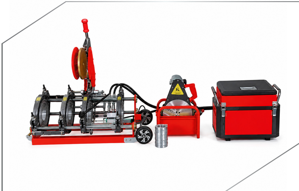
دستگاه جوش پلی اتیلن CNC 250 چهار فک RSCO مدل HPCD-250
