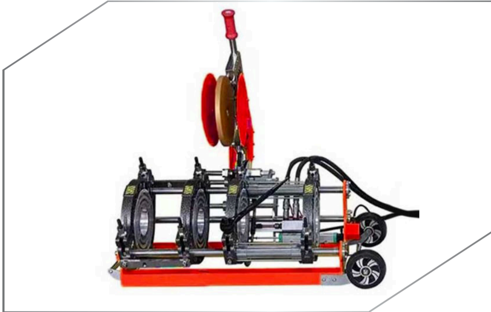
دستگاه جوش پلی اتیلن CNC 315 چهار فک RSCO مدل HPCD-315
