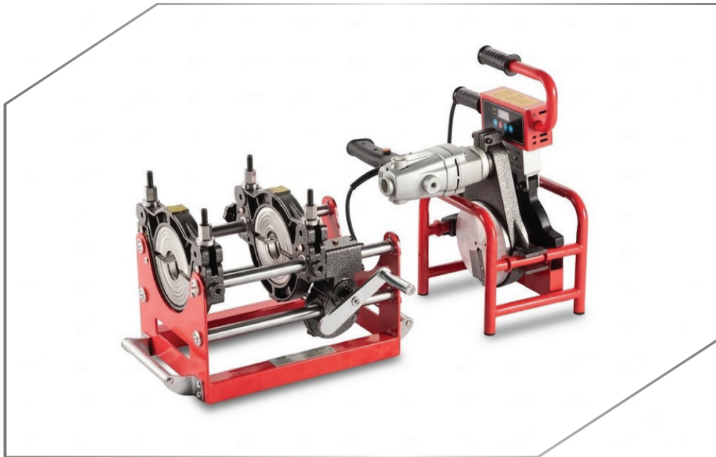
دستگاه جوش پلی اتیلن دستی 200 دو فک RSCO مدل MD2-200
