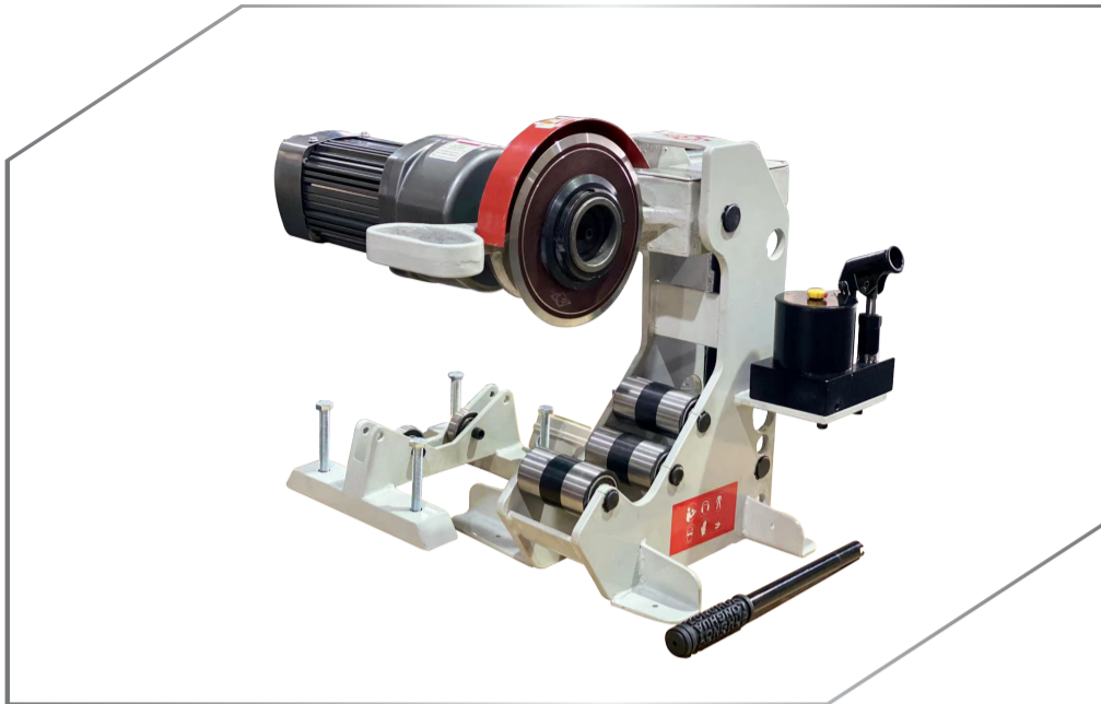
لوله بر برقی صنعتی RSCO مدل BPC820
