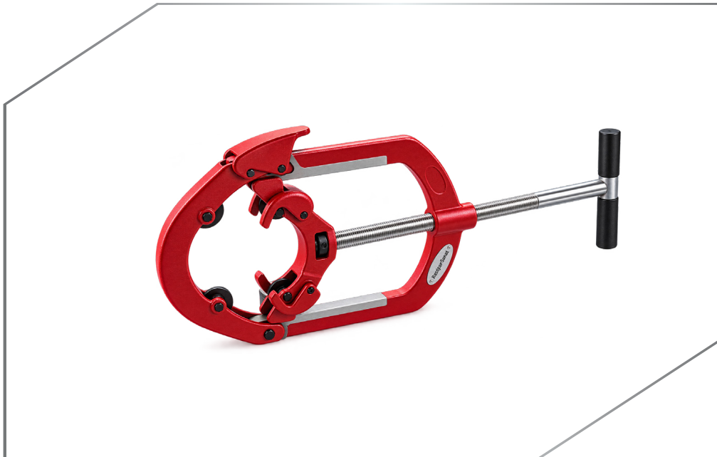
لوله بر دستی 8 اینچ 4 تیغ RSCO مدل CPM84
