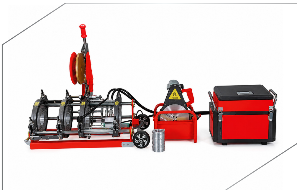
دستگاه جوش پلی اتیلن CNC 200 چهار فک RSCO مدل HPCD-200
