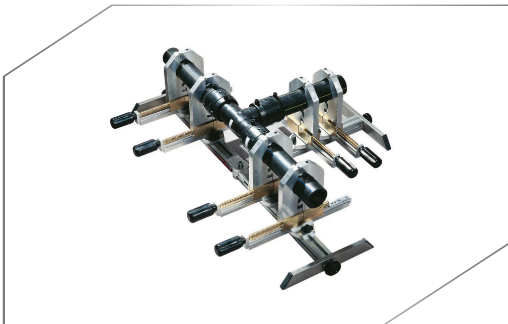
مولتی کلمپ پلی اتیلن 160 میلیمتر RSCO مدل PECM161
